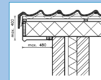
Windveer overstek
