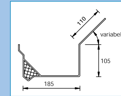
C-goot
