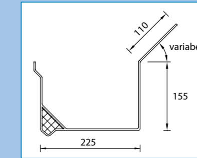
A-goot
