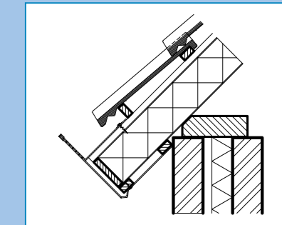
V-goot
